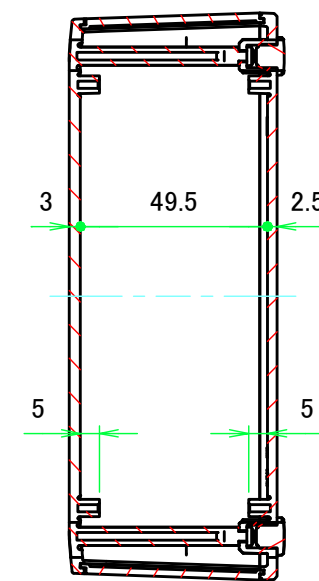
A-A ( 1 : 2 )
